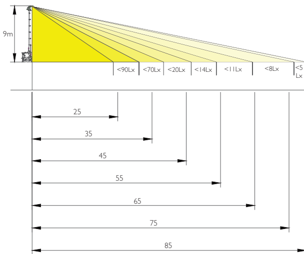
MIDSTREAM Mobile Tower1台における照明可能範囲
