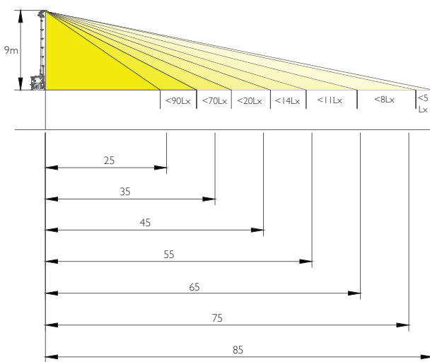
MIDSTREAM Mobile Tower1台における照明可能範囲
